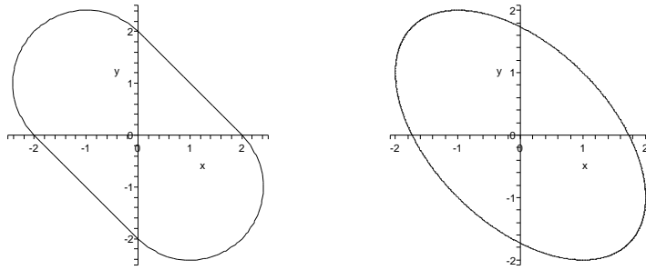
(d) Unit circle of the 1-HH-norm (e) Unit circle of the 2-HH-norm
